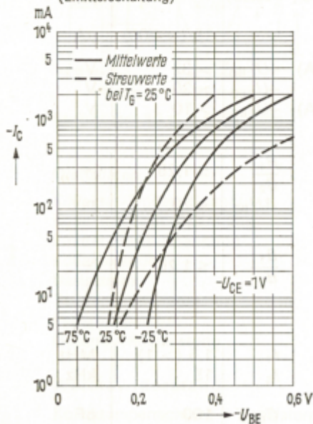
Kollektorstrom I_C = f(U_{BE}) -U_{CE} = 1 \text{ V}; \text{ Streukurven (Emitterschaltung)}
